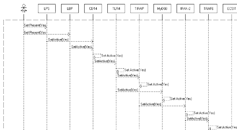
Abbildung 10: TLR 4 – Ausschnitt aus einem LSC-Diagramm.
