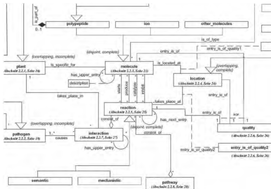
Abbildung 2: Konzeptionelles Schema für die PathoPlant-Datenbank (Teilansicht).
