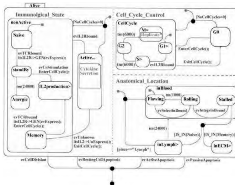
Abbildung 5: Statechart-Modell der T-Zellen-Aktivierung (N.Kam).
