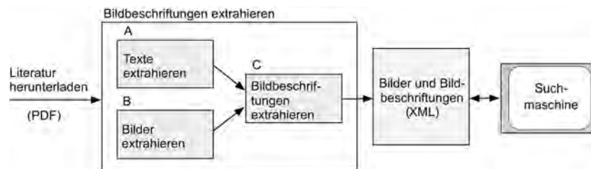
Abbildung 7: Datenfluss.
