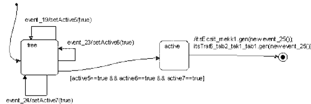
Abbildung 12: TLR4 – Statechart-Diagramm.
